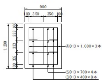
電動パワーユニット基礎 平面図
