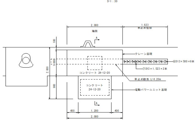
電動パワーユニット基礎 平面図
